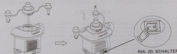
Abb. (6): ANSCHLIESSEN DER DÜSEN
